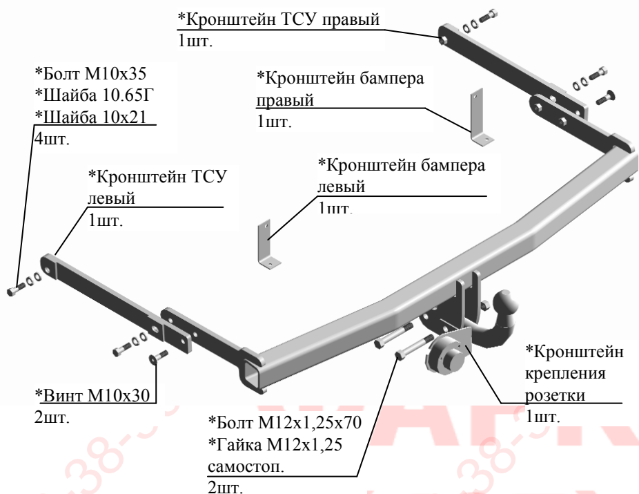
Рис.1 Тягово-сцепное устройство 6030
